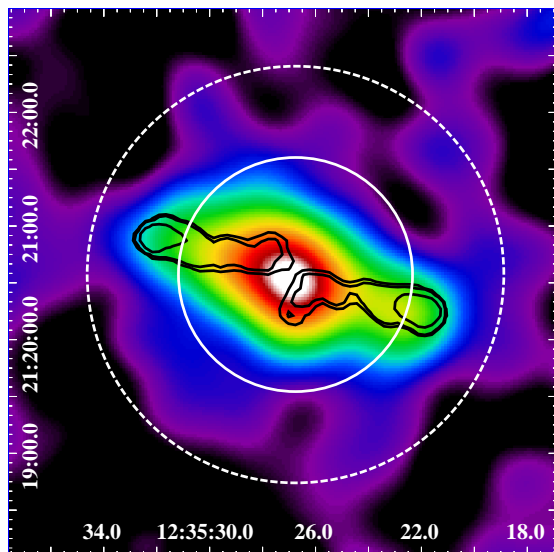
FIG. 12.— 3C 274.1
