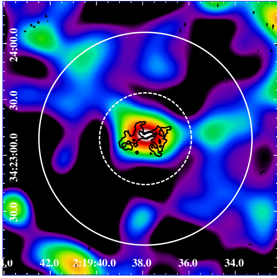
FIG. 9.— 7C 0219+3423
