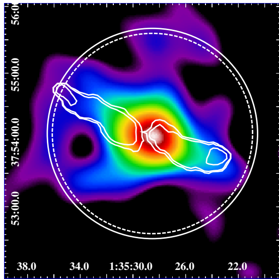
FIG. 11.— 3C 46
