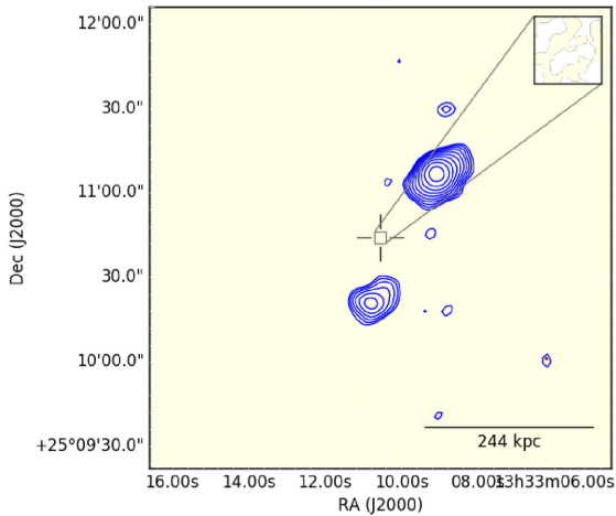
(ag) J133309.94+251045.2
