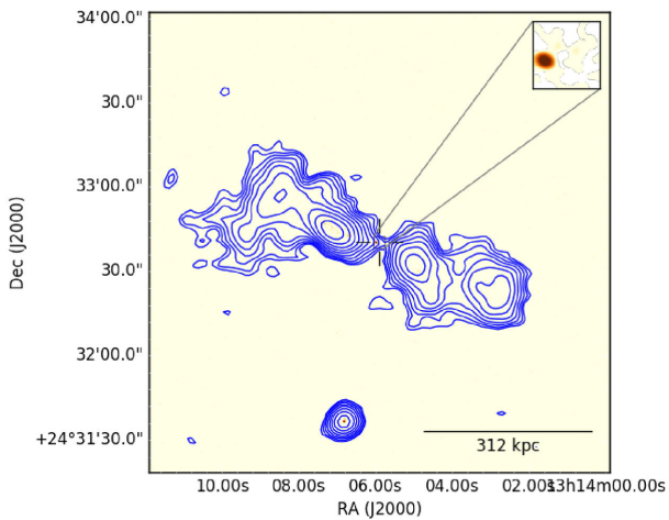
(u) J131405.16+243234.1
