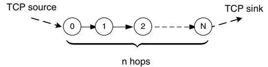
Fig. 1. String topology
